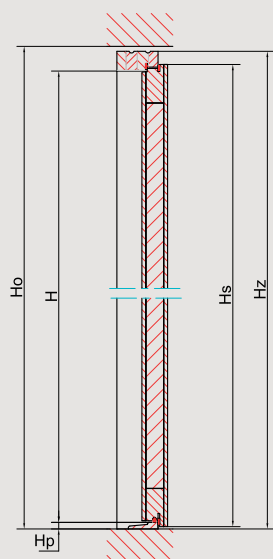
PRZEKRÓJ PIONOWY SKRZYDŁA Z OŚCIEŻNICĄ
